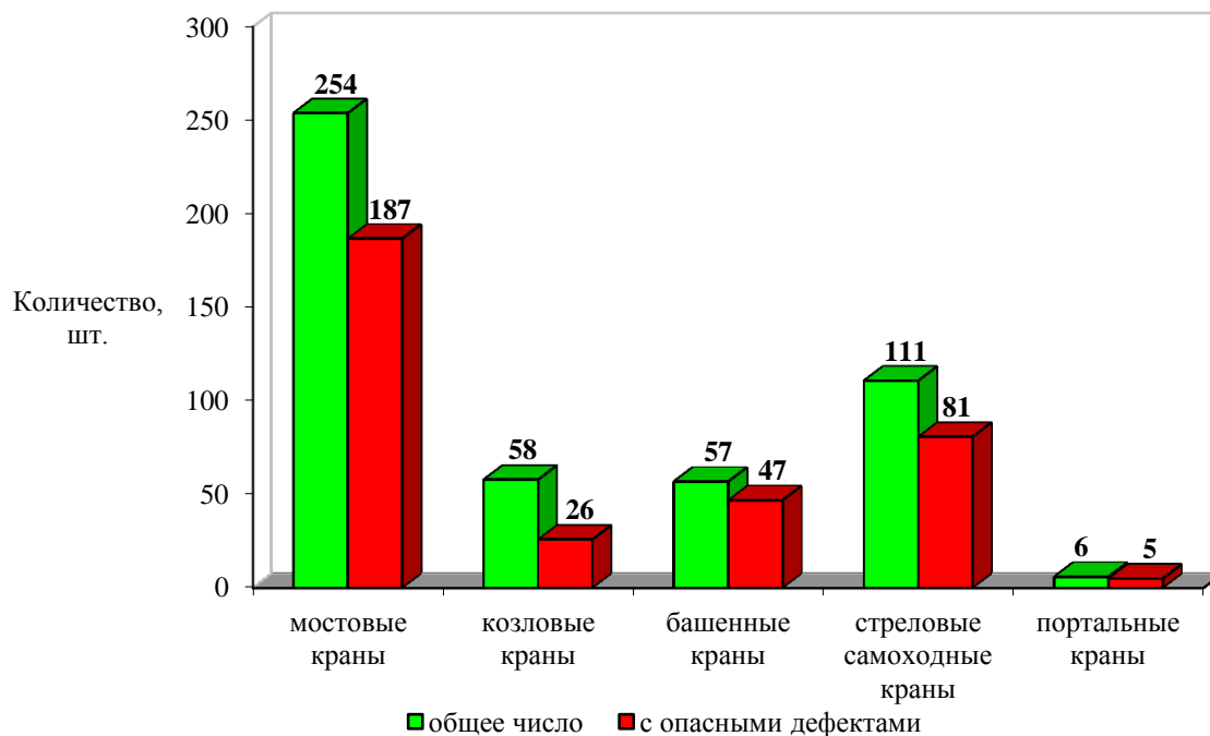
Рис. 1. Соотношение кранов с опасными дефектами к общему числу (по типам кранов).
